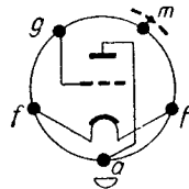
Sockelschaltenschema
