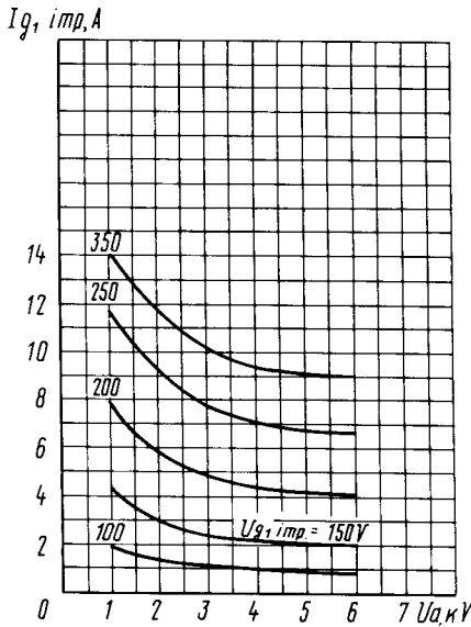
Усредненные импульсные характеристики: U_{g2} = 2 кВ Averaged Peak Characteristic Curves: U_{g2} = 2 kV
