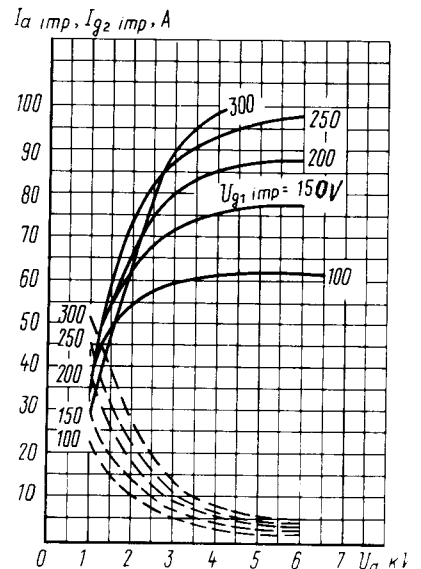
Усредненные импульсные характеристики: U_{g2} = 2,5 кВ; — анодные; - - - анодно-сеточные (по сетке второй) Averaged Peak Characteristic Curves: U_{g2} = 2,5 kV; — anode; - - - anode-grid 2
