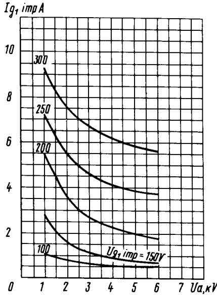
Усредненные импульсные характеристики: U_{g2} = 2,5 кВ Averaged Peak Characteristic Curves: U_{g2} = 2,5 kV
