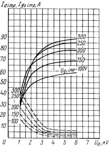
Усредненные импульсные характеристики: U_{g2} = 2 кВ; — анодные; - - - анодно-сеточные (по сетке второй) Averaged Peak Characteristic Curves: U_{g2} = 2 kV — anode; - - - anode-grid 2
